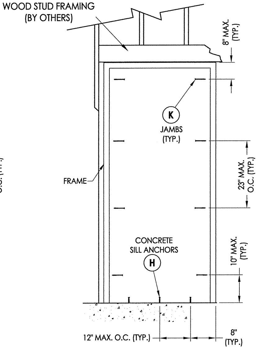
FRAME ANCHORING Wood Stud
